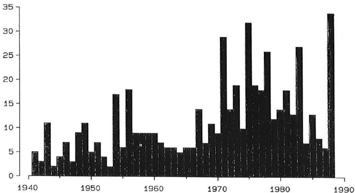
Antal stormdygn, d.v.s. dygn då medelvinden nått minst 21 m/s vid Kullen under åren 1941-1988.
