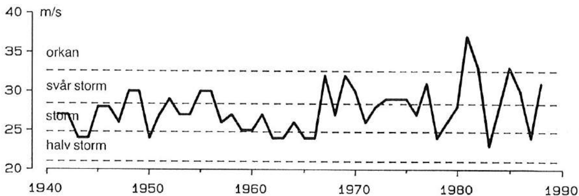
Högsta medelvind per 10 minuter (m/s) som noterats vid Kullen under åren 1941-1988.
