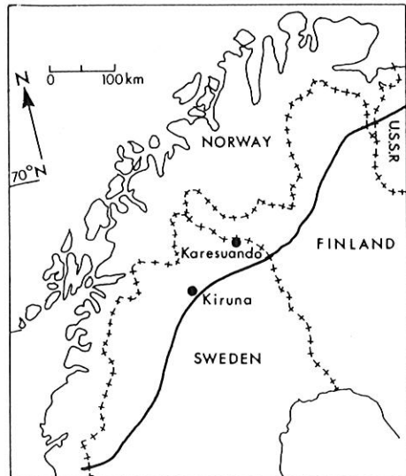
Figur 1. Den osammanhängande permafrostens sydostgräns (hel-dragen linje) sammanfaller helt med gränsen för granskogens utbredning. Efter A. Rapp (1982).
